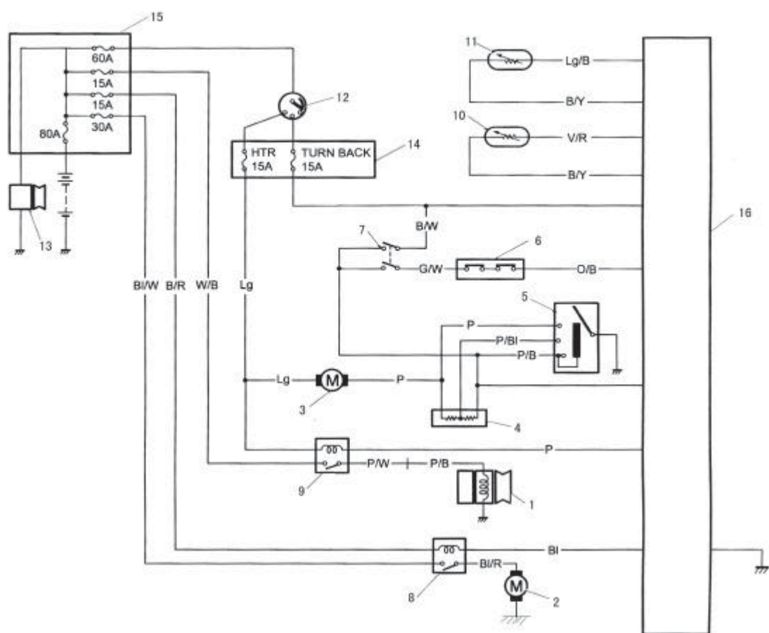
电路图
